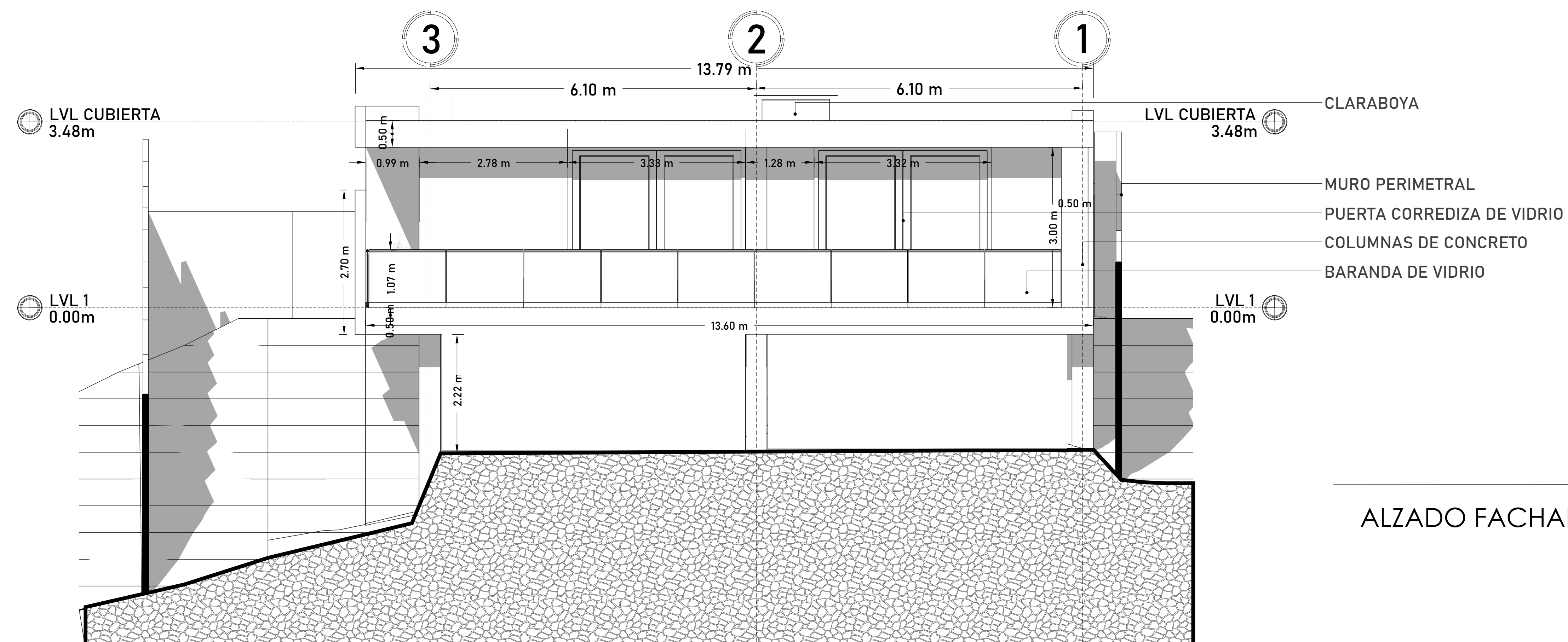
ALZADO FACHADA LATERAL
