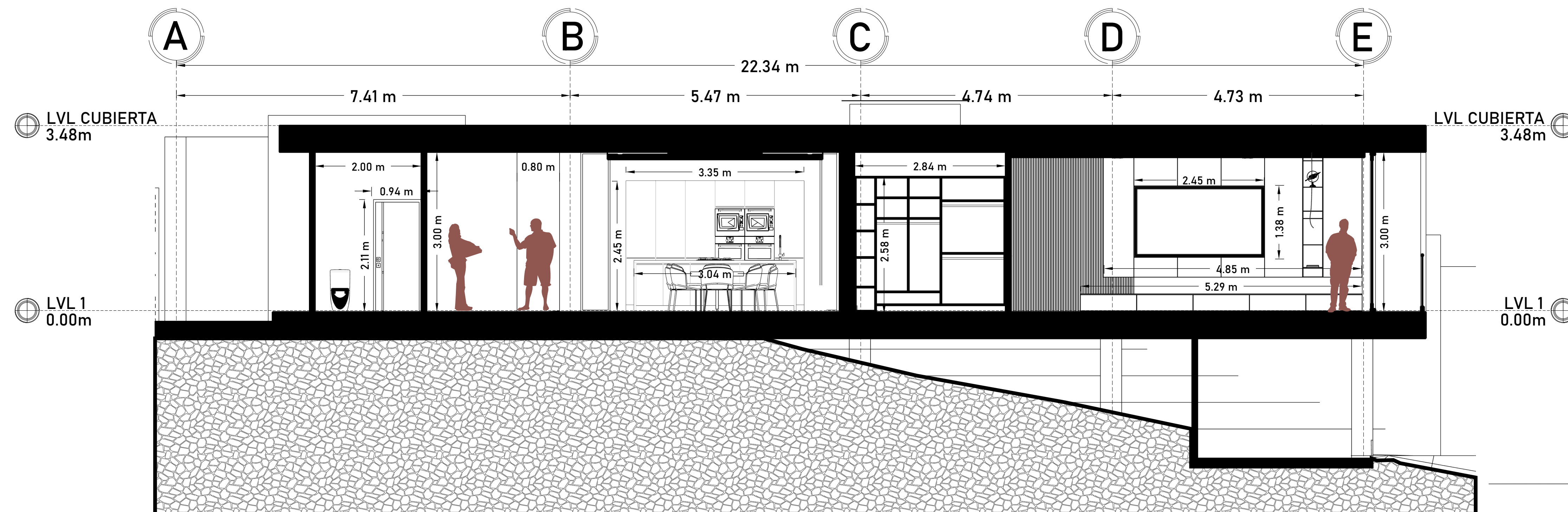
CORTE LONGITUDINAL
